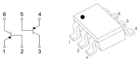
SOT-363
